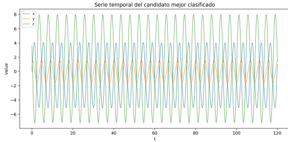
Figura 11. Series temporales de las variables x(t) , y(t) y z(t) del candidato en régimen de estado transitorio final y estable.
