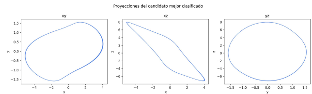
Figura 10. Proyecciones geométricas en los planos xy , xz y yz para el atractor candidato fraccionario.
