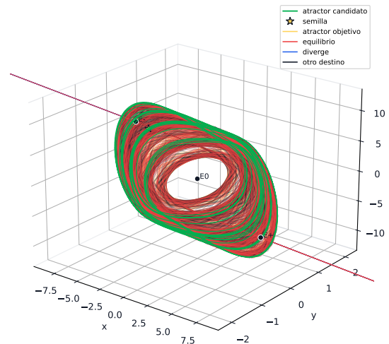
Figura 4. Sondeos de ocultación desde vecindades de los equilibrios. La ausencia de trayectorias clasificadas como TARGET apoya la clasificación del régimen como candidato numérico a atractor oculto.
