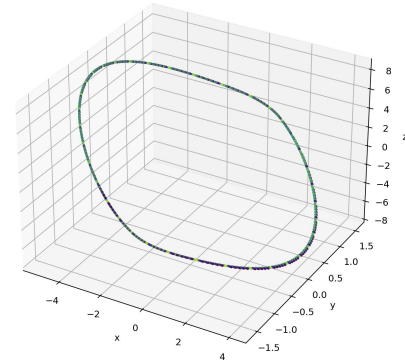
Figura 9. Espacio de fases 3D para el candidato centered_machado_mu2 en Chua fraccionario ( q = 0.9998 ) integrado con C EFORK-3.
