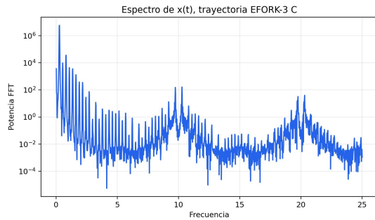
Figura 12. Espectro de potencia FFT de la señal x(t) que muestra el carácter caótico y de banda estrecha del atractor.
